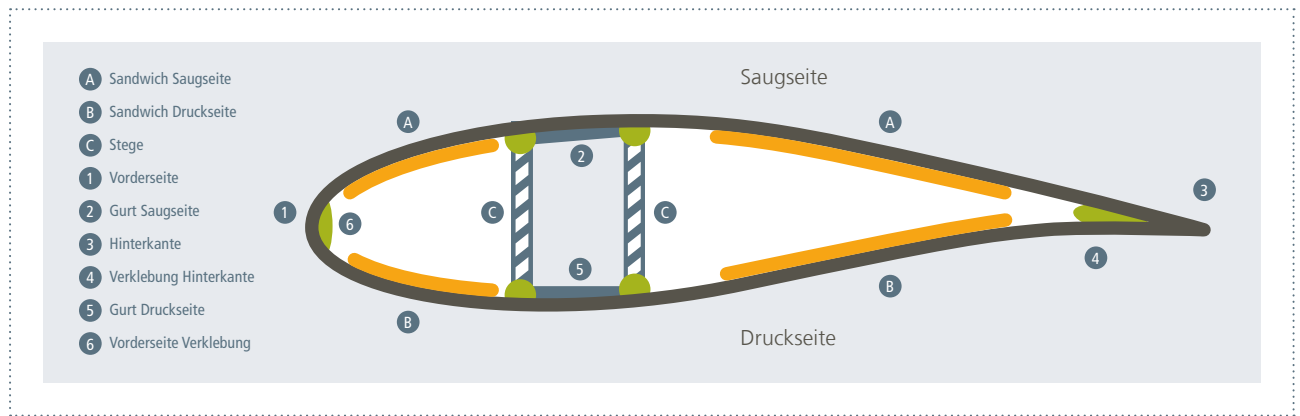
Abbildung 2: Schematischer Aufbau eines Rotorblattes
